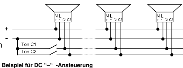
Beispiel für DC „-“ -Ansteuerung
