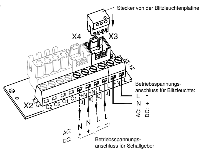
getrennter Anschluss von Blitzleuchte und Schallgeber
