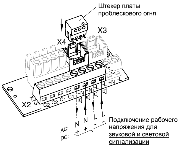
Общее подключение звуковой и световой сигнализации (вид поставляемого изделия)
