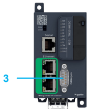
3 TM251MES controller
